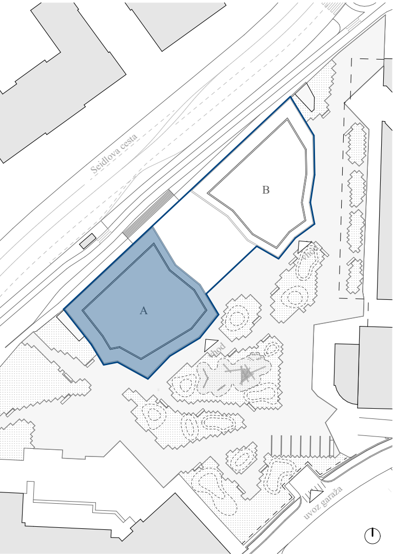
Položaj situacija- A blok, M 1_1000
