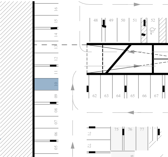
Položaj parkirnih mest- 10, klet -2, M 1_500
