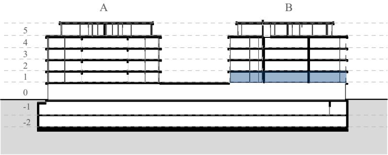
Položaj nadstropja - 1.nadstropje, M 1_1000
