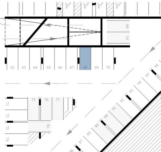
Položaj parkirnih mest- 68, klet -2, M 1_500
