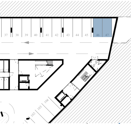
Položaj parkirnih mest-46 in 47, klet -2, M 1_500
