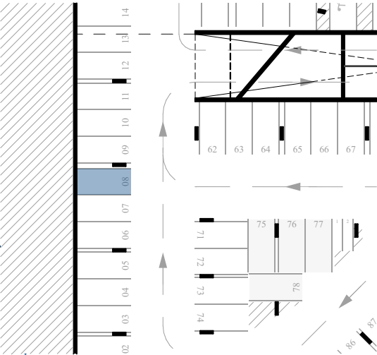
Položaj parkirnih mest- 8, klet -2, M 1_500
