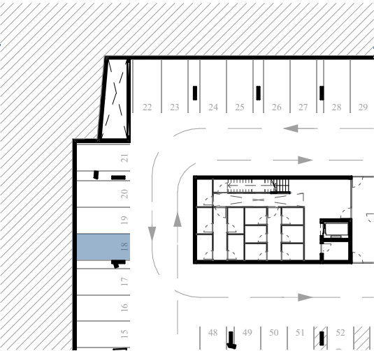
Položaj parkirnih mest- 18, klet -2, M 1_500
